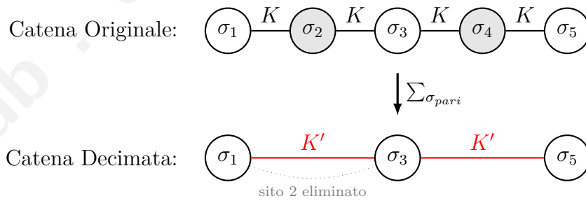
Figura 24.1: Rappresentazione grafica della decimazione: eliminazione dei siti pari e rinormalizzazione dell'accoppiamento tra i siti rimanenti.
