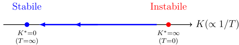
Figura 24.2: Diagramma del flusso di rinormalizzazione per il modello di Ising 1D. Ogni accoppiamento finito K fluisce verso il punto fisso stabile a K = 0 (temperatura infinita), indicando l'assenza di una fase ordinata a temperatura finita.
